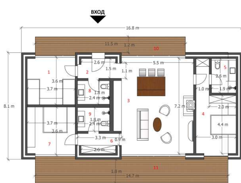
РАЗПРЕДЕЛЕНИЕ ±0.00
